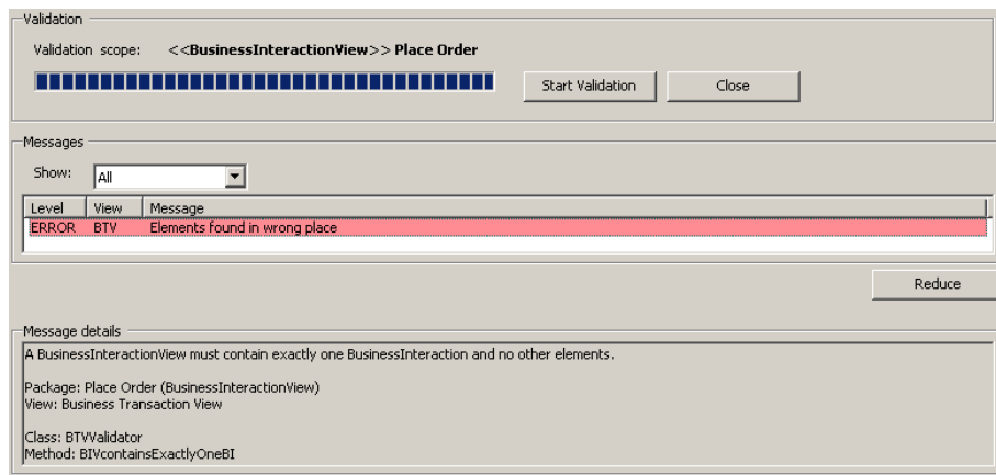
Fig. 3. UMM Validator
